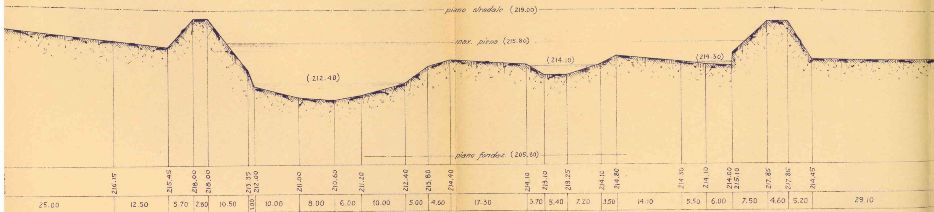
— Sezione dell'alveo sull'asse del nuovo ponte —
